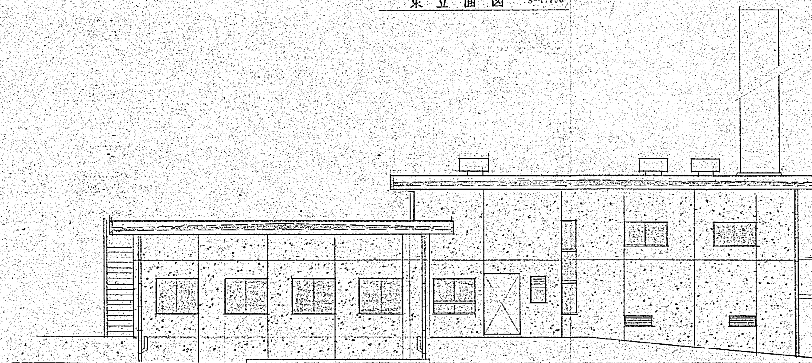
東立面図 S=1:100
