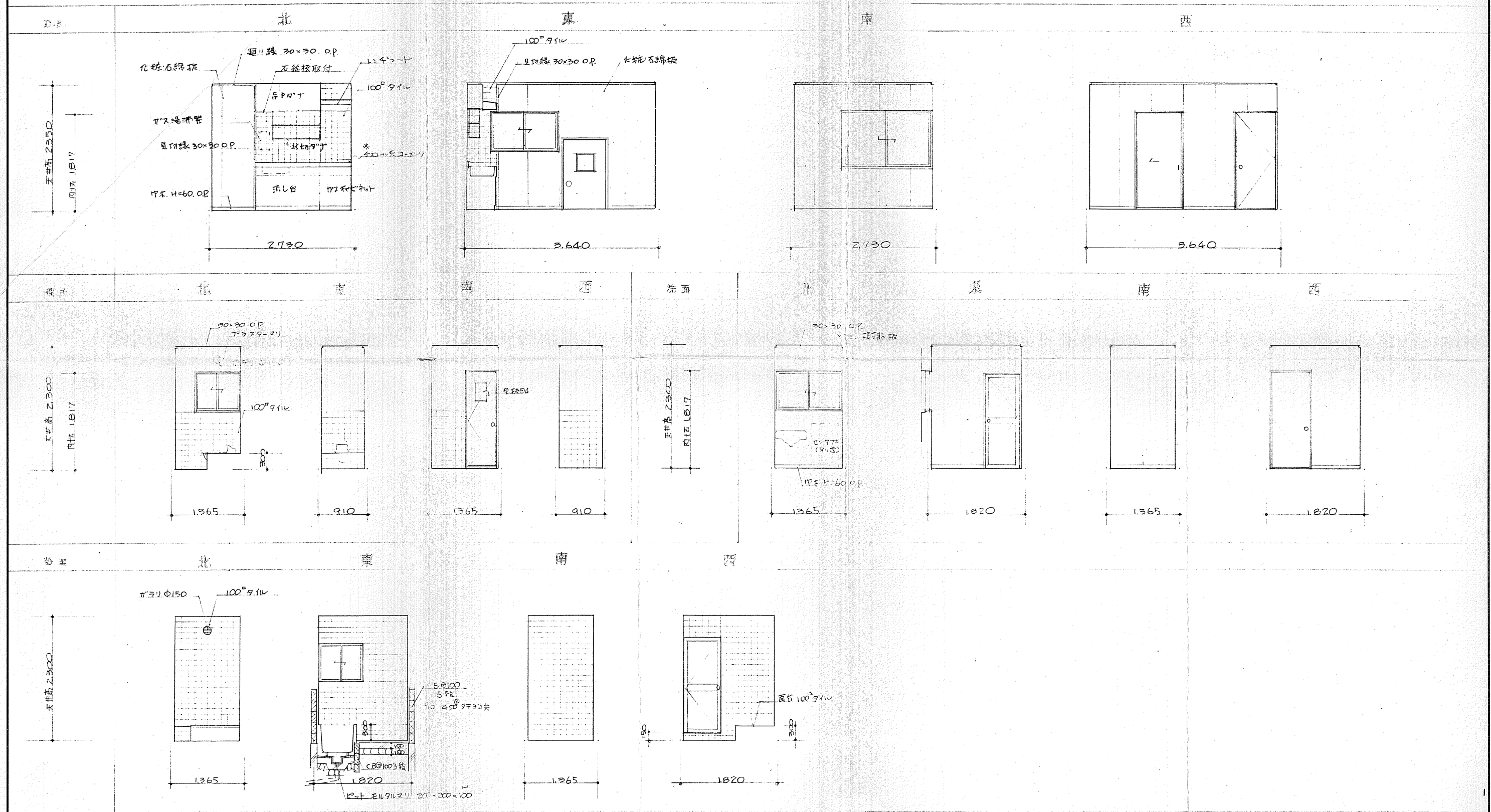
展開図 2 S. 1/50
