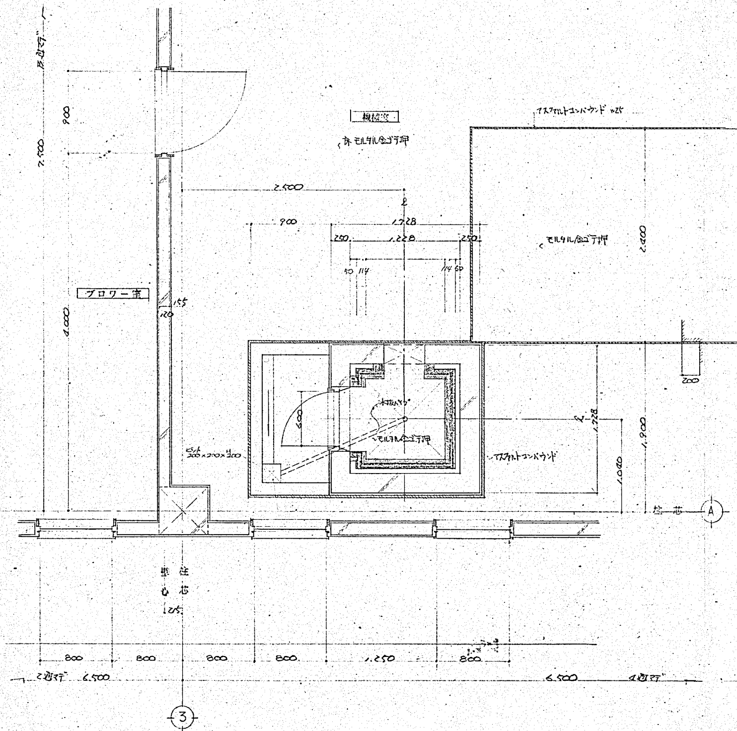
平面詳細図 S=1:50
