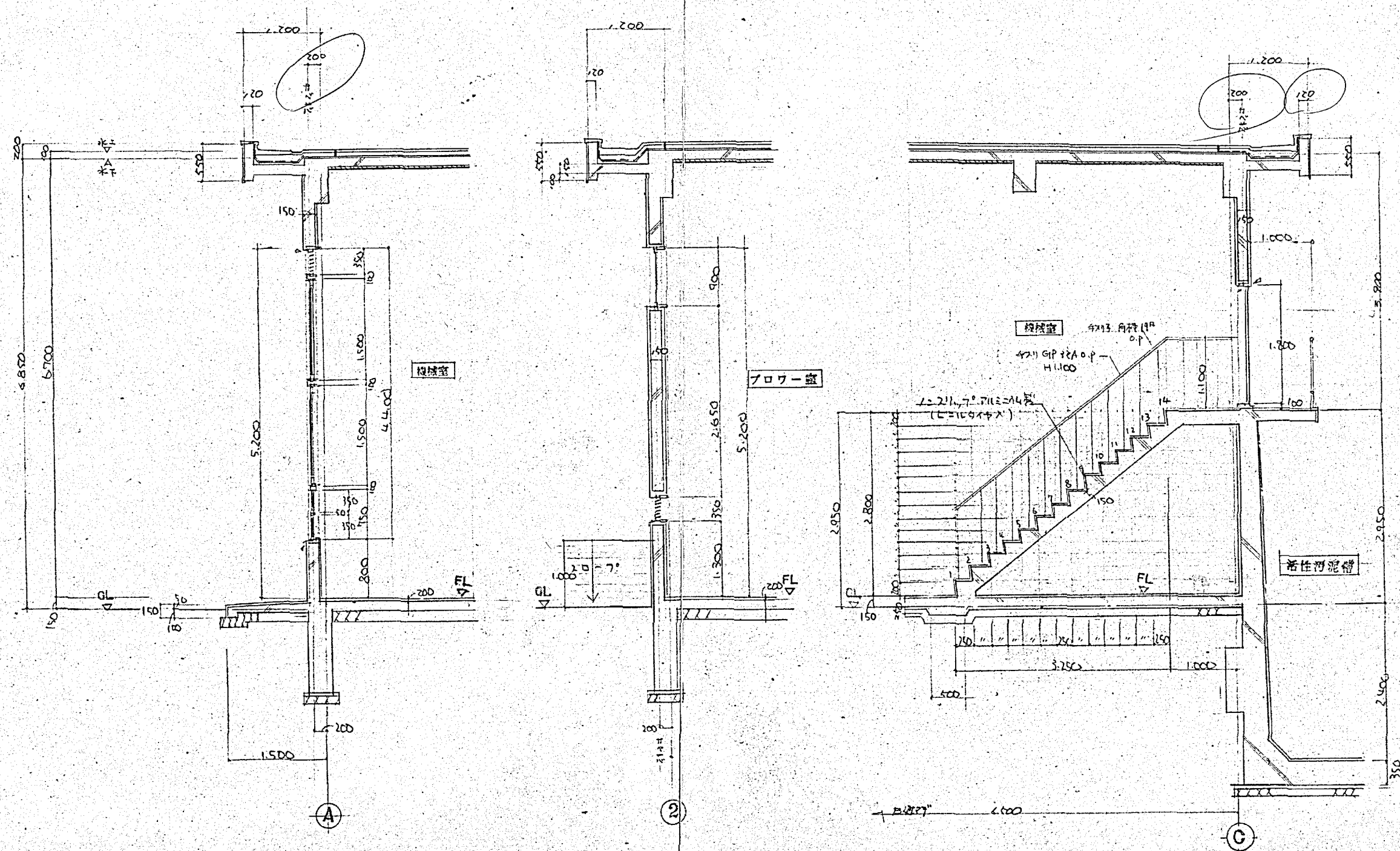
矩計図 S=1:50
