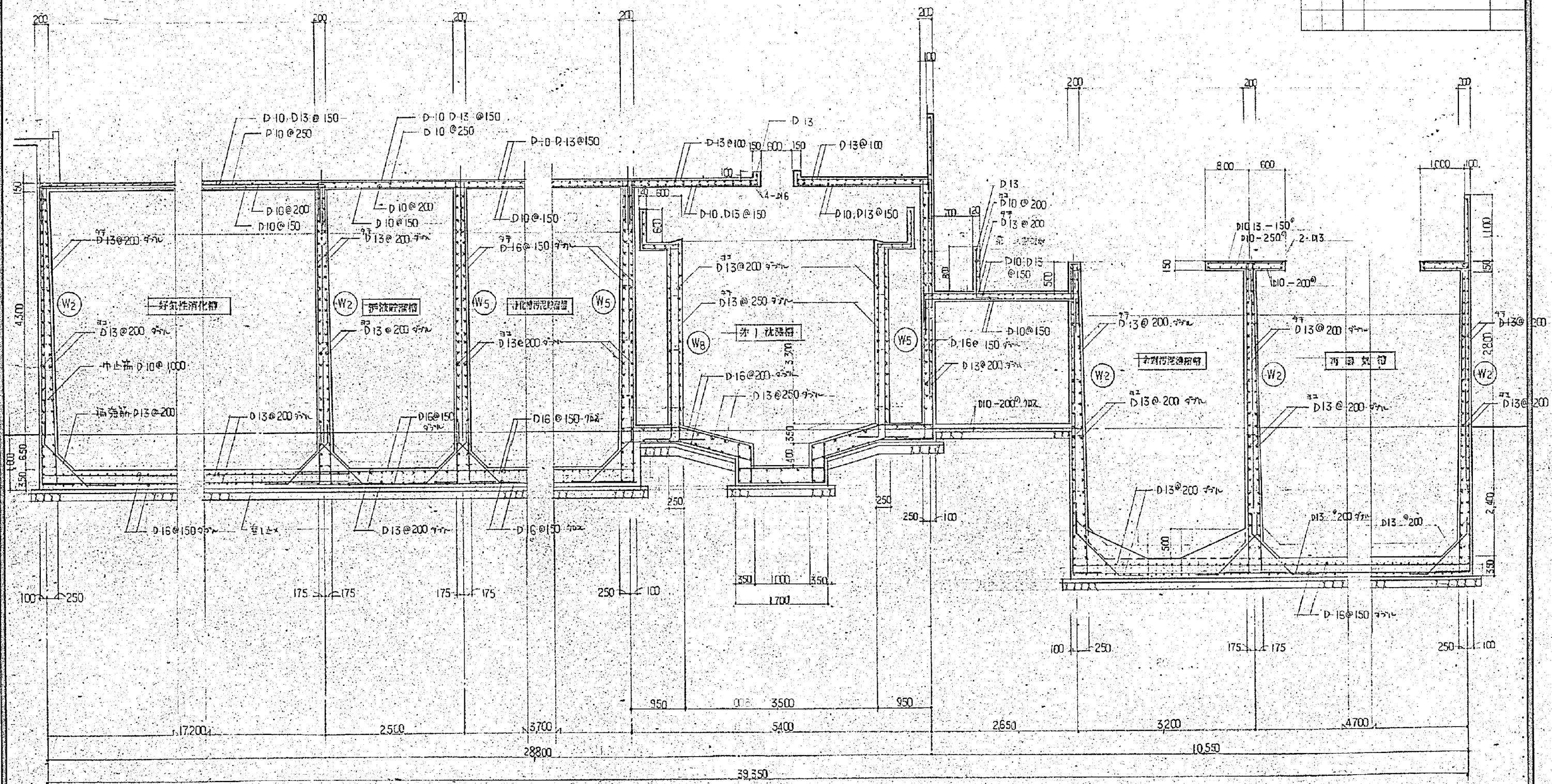
断面配筋図 S-1:50
