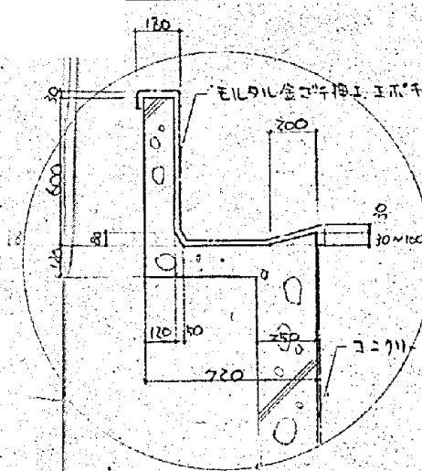
A部断面詳細図 S=1/20
