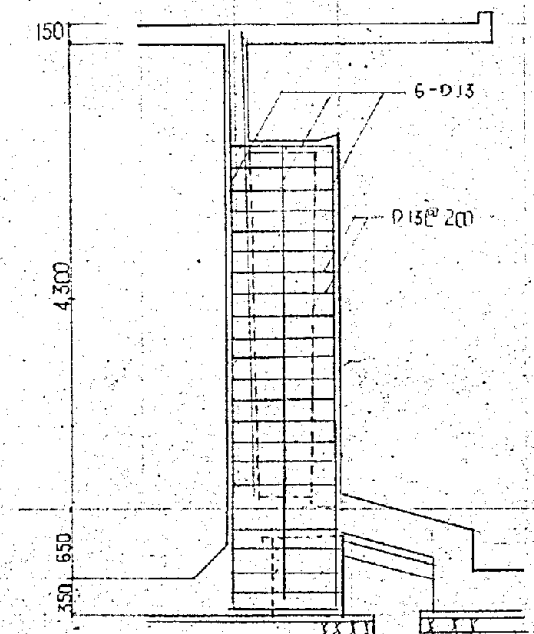
② 断面配筋図 S=1:50
