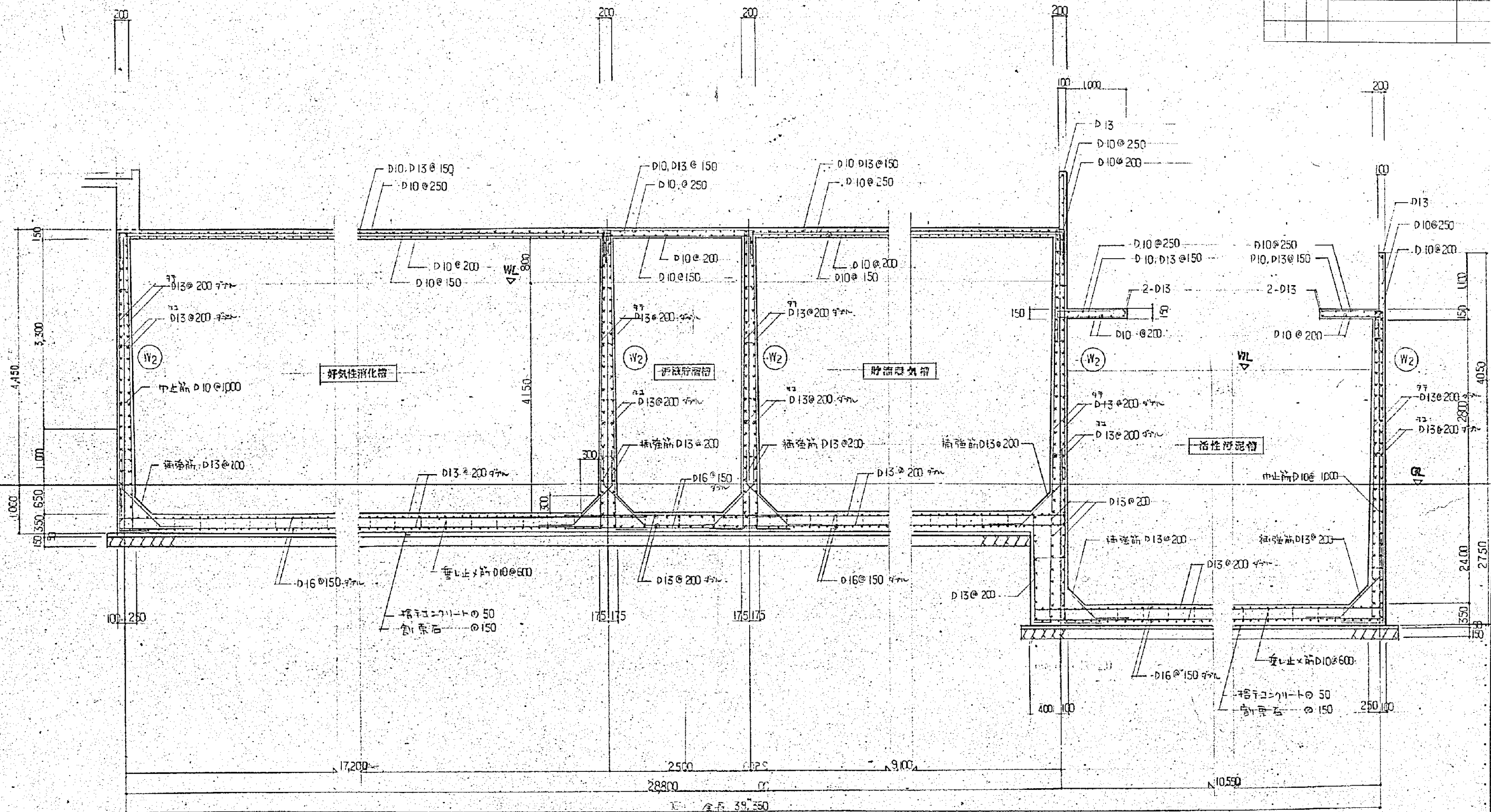
断面配筋図 S=1:80
