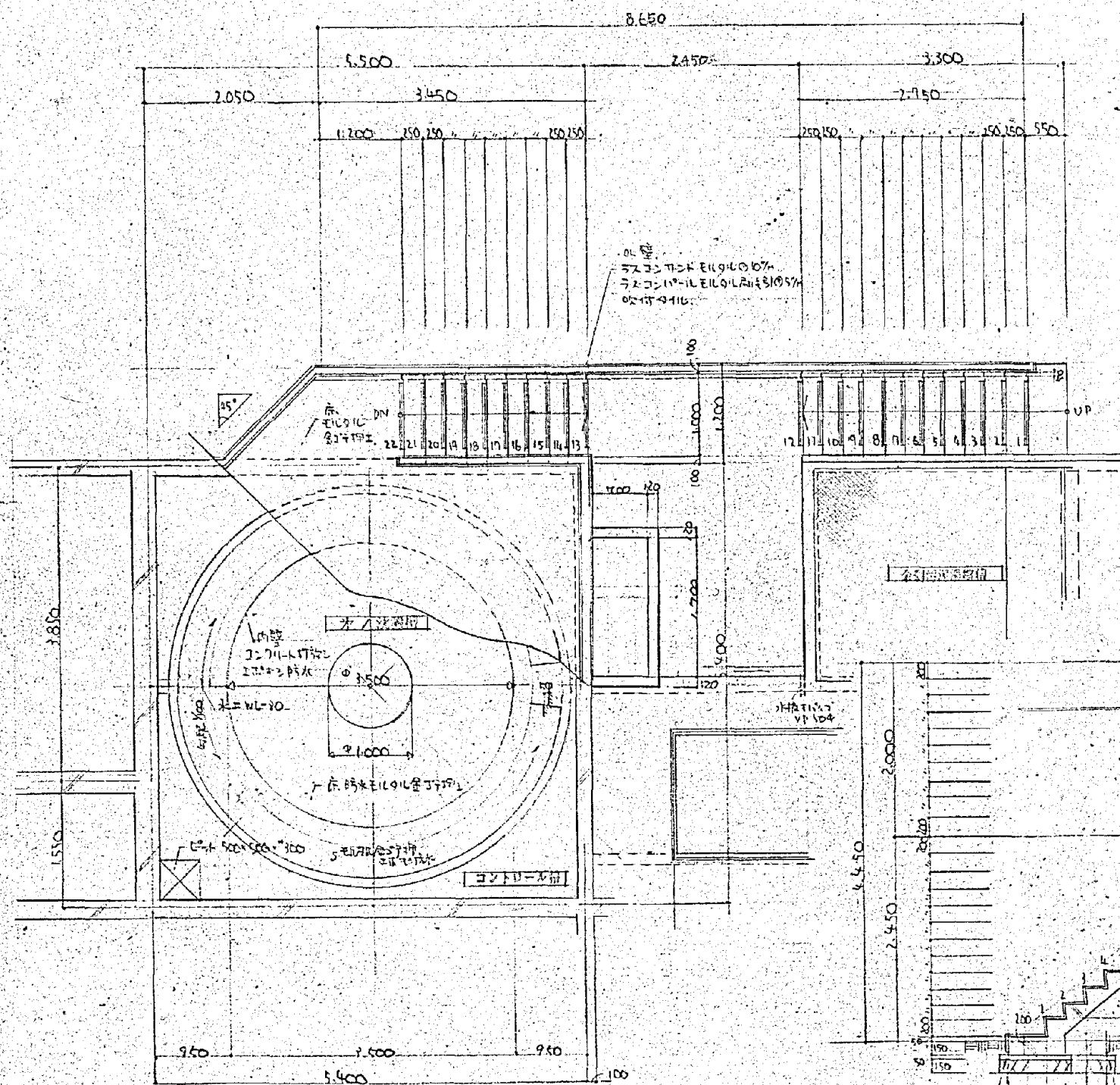
第1処理室 & 階段 平面図 S=1/50
