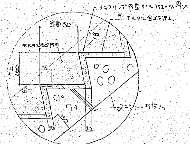
A部 断面詳細図 S=1/10
