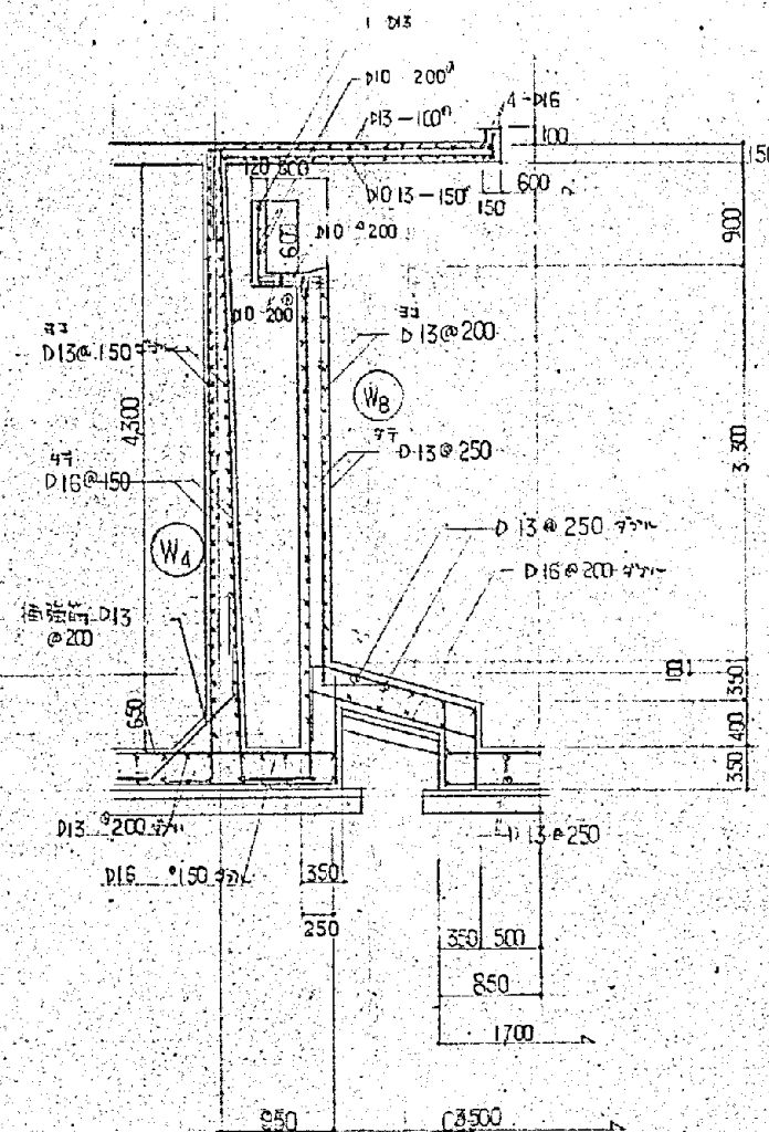
① 断面配筋図 S=1:50
