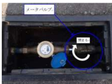
ボールバルブタイプ 90度横にまわす
