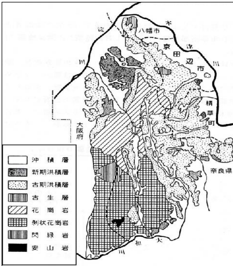
■生駒山地の地質図
