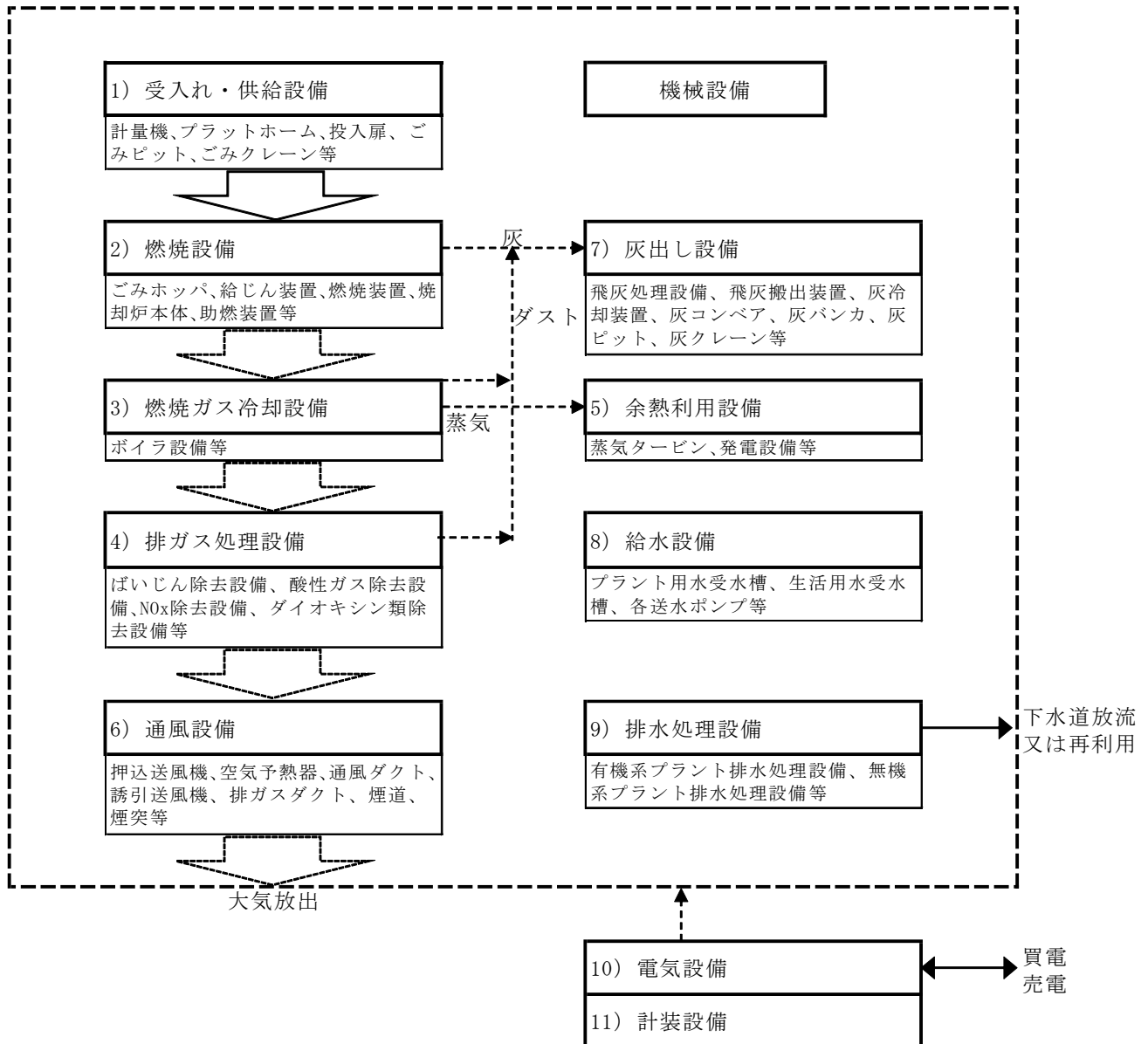
【焼却処理設備の構成】
