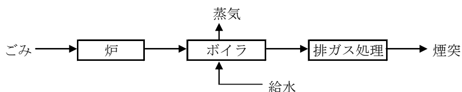
【廃熱ボイラによる熱回収概略フロー】
