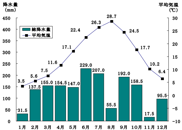
気象概況 (平成22年)
