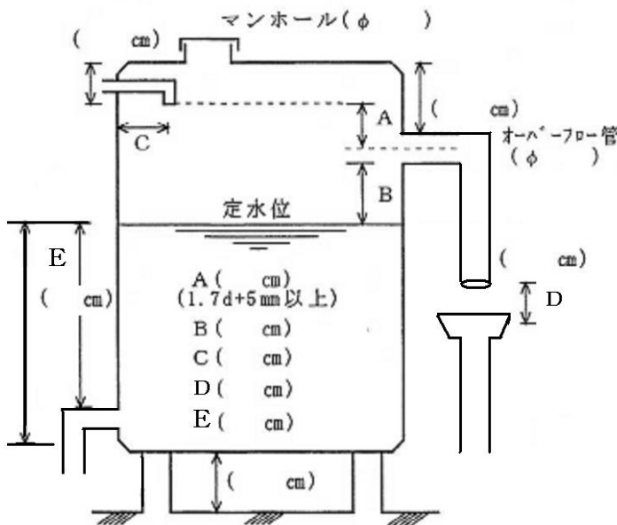
受水槽の構造図
